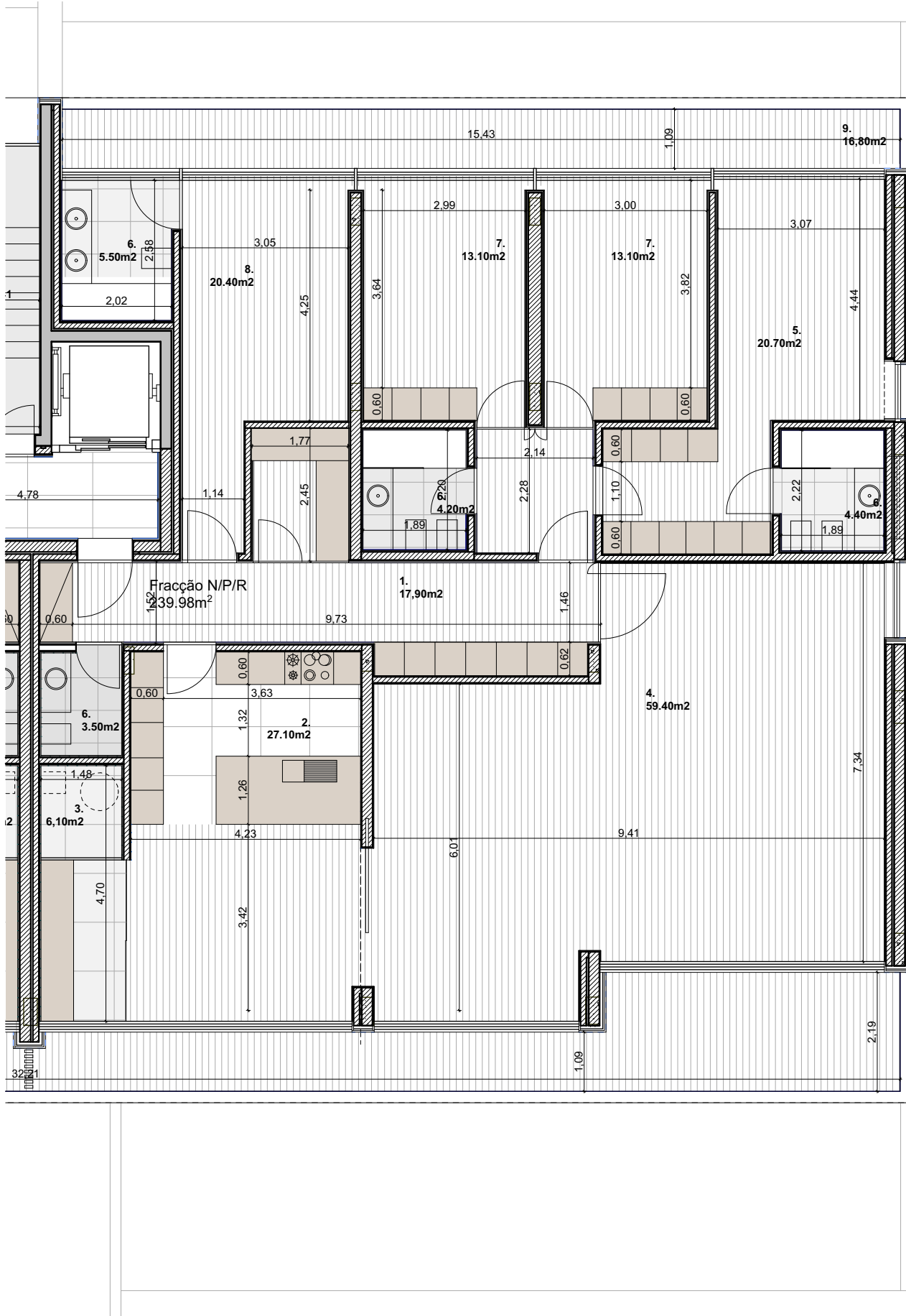
T4 (Piso Tipo)
